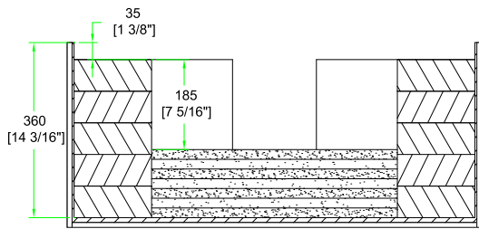
A-A VIEW
