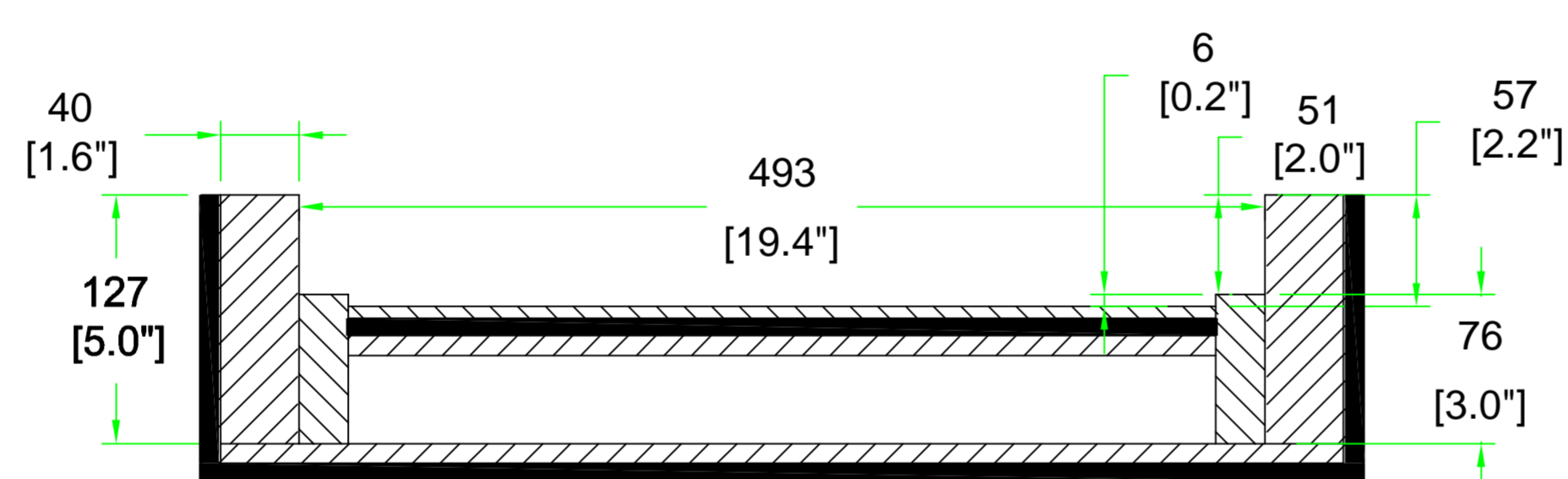
A-A VIEW
