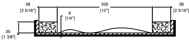
A-A VIEW
